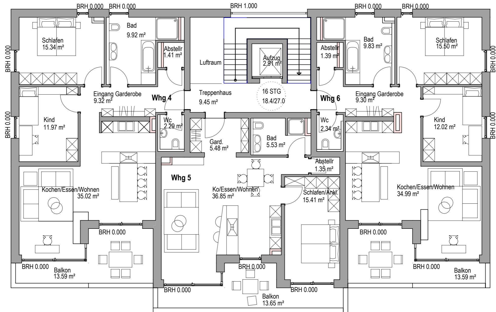
Obergeschoss Haus 22/1
